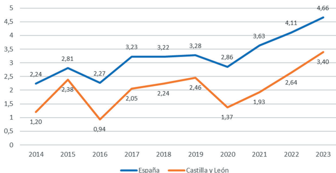
Figura 1.–Incidencia de Legionelosis en España y Castilla y León (tasas por 100.000 habitantes). Años 2014-2023.
